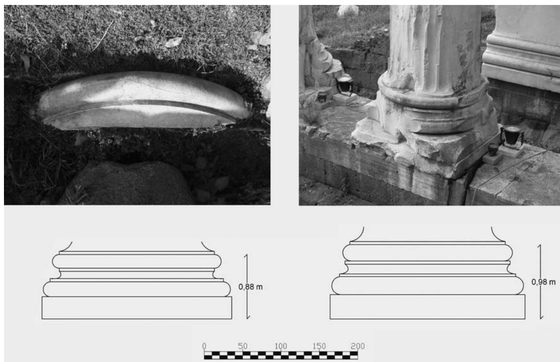
Figura 15. Comparación de las basas del templo de Claudio y de Mars Ultor .
