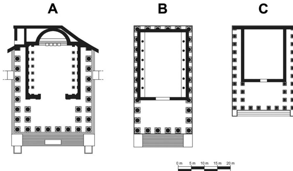
Figura 21. Plantas comparadas del templo de: A) Mars Ultor . B) Claudio en Roma. C) Claudio en Camulodunum .
