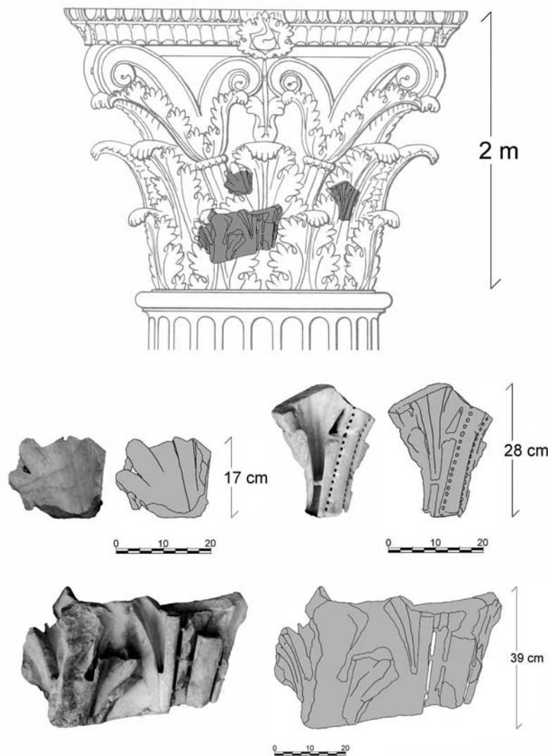
Figura 16. Reconstrucción de las medidas de los capiteles del Claudianum .
