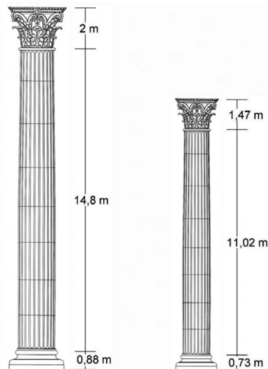
Figura 18. Comparación de las medidas de las columnas del templo de Claudio y del propileo de acceso al temenos.
