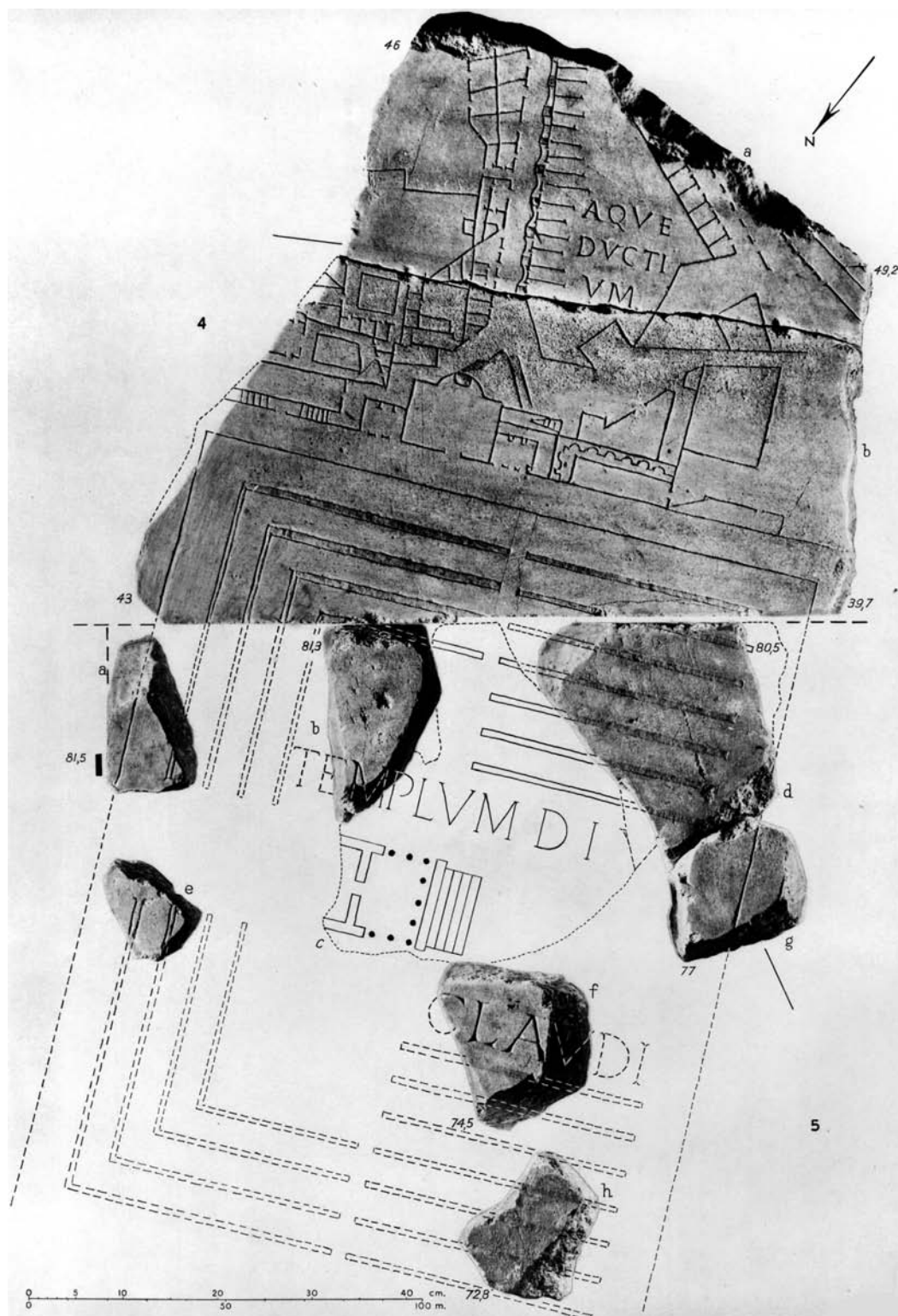
Figura 1. Restitución de la planta del Claudianum en base a los fragmentos de la FUR (Carettoni, Colini, Cozza, Gatti 1960, Tav. XVI).
